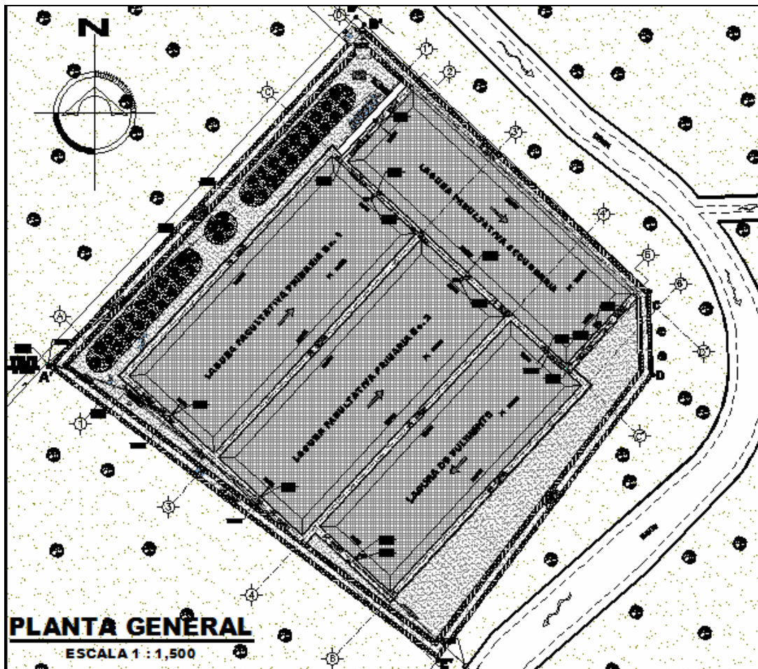
Figura 3. Arreglo de planta del sistema de tratamiento
